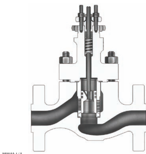
图2. Fisher HPD 阀门组件 (NPS 2 至 NPS 6)
