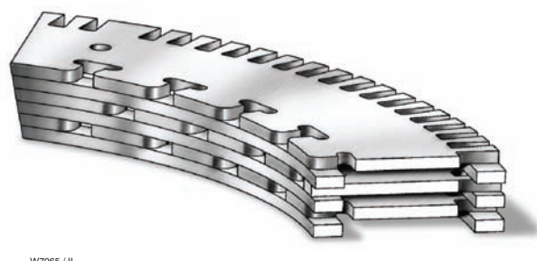
图3. 用于 Fisher HP 阀门的典型 WhisperFlo 内件
