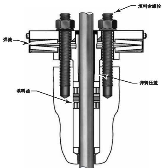
典型使用石墨 ULF 填料的 HIGHT-SEAL 填料函系统
