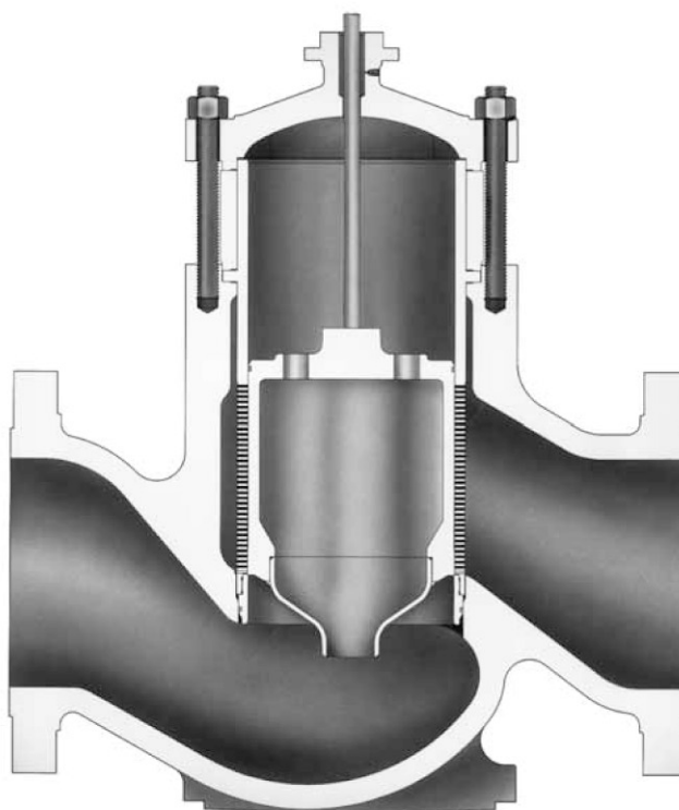
图4. 配阀帽隔离段和Whisper Trim® III 阀笼的特殊EWT-2 阀门
