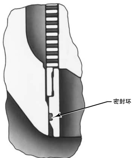
座环密封详图
