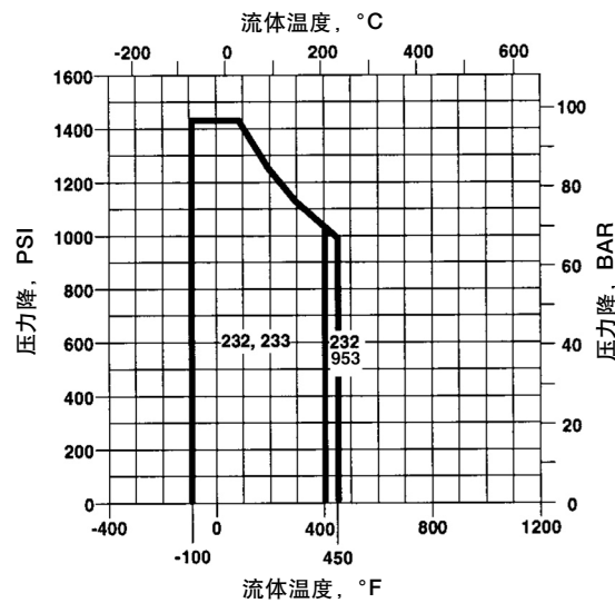
用于 600 磅级 CF8M (316 不锈钢) 阀体标准金属座环<1>
