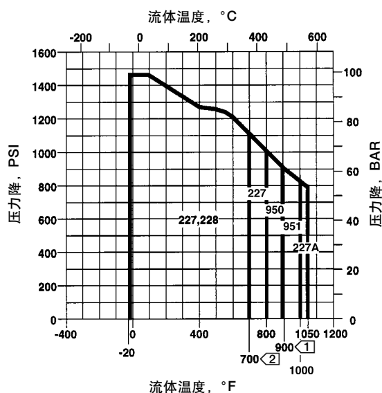
用于 600 磅级 WC9 铬钼阀体标准金属座环
