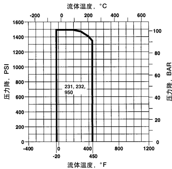
用于 600 磅级 WCC 钢阀体标准金属座环<1>
