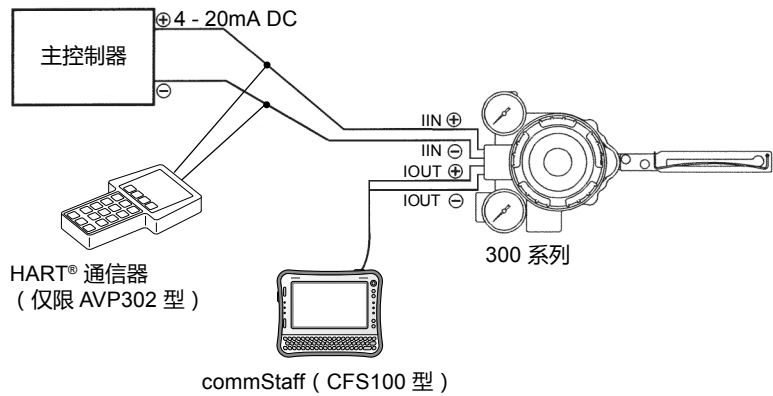
图 1. 通用电-气动定位器 ( AVP300/302 型 )
