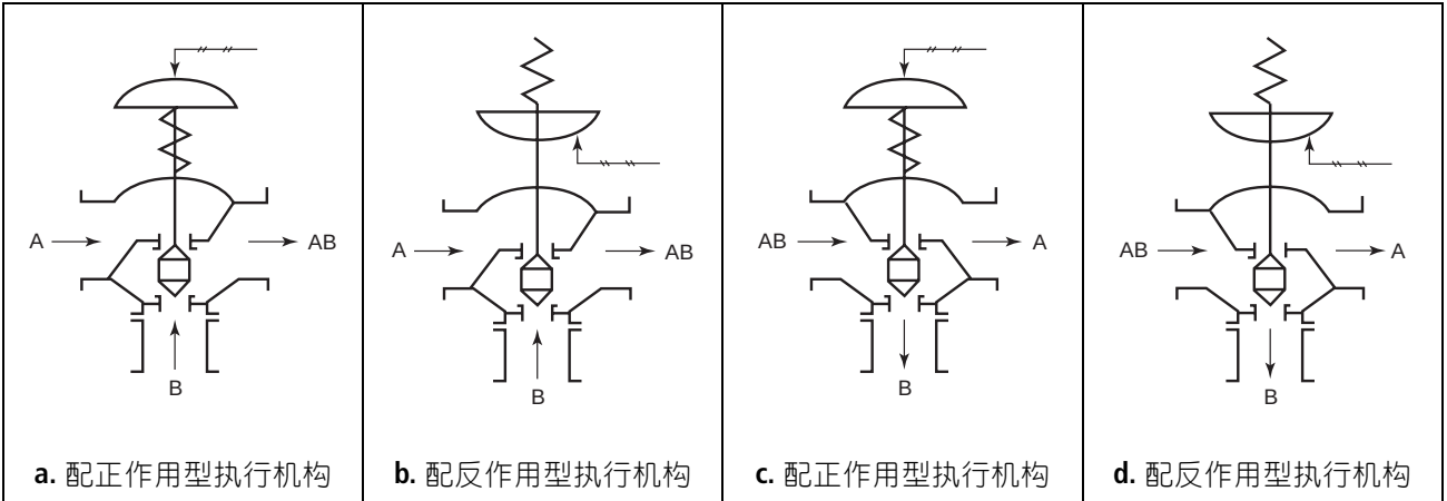
图 3 阀作用
