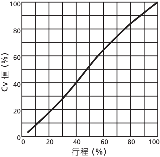
图 2 流量特性
