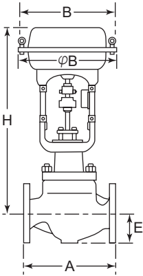
图 4 法兰间距和其他尺寸
