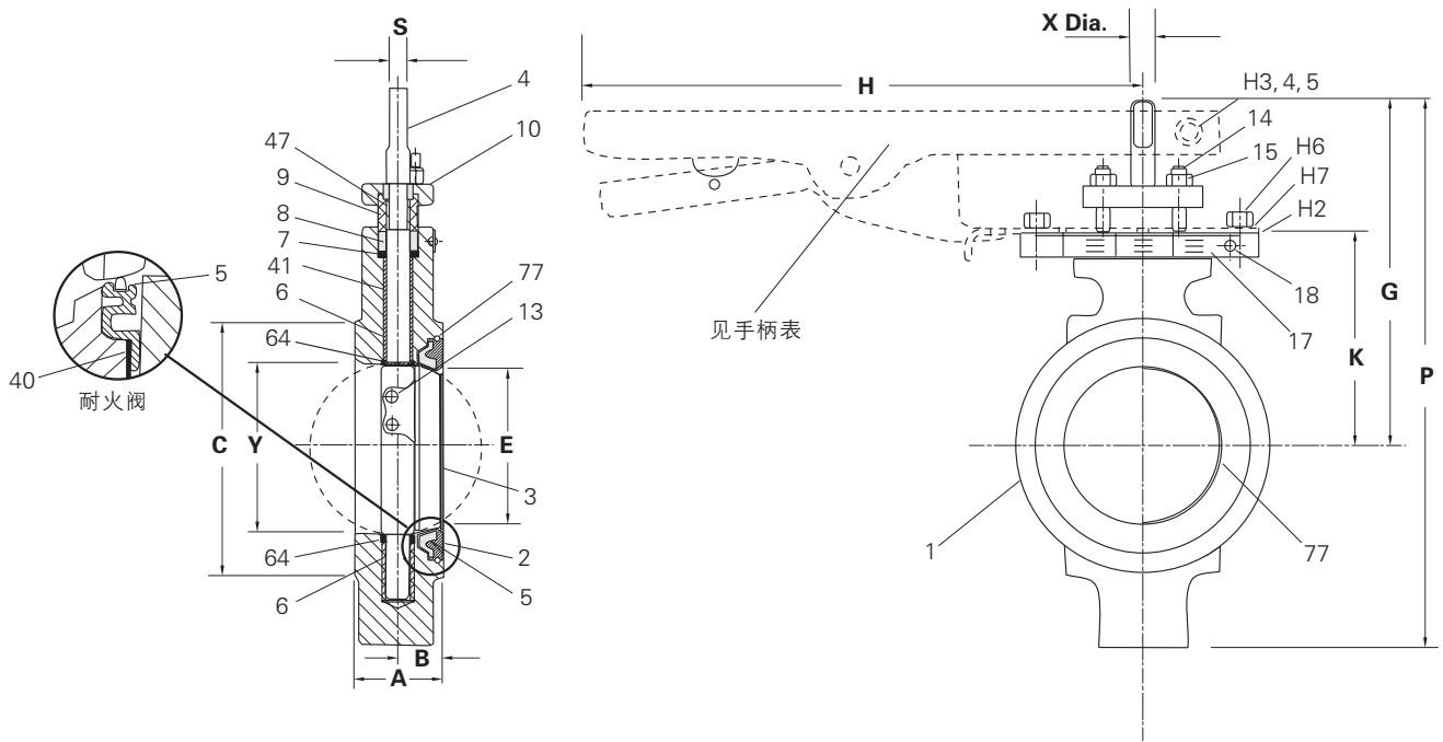
2-1/2" ~ 12" ( DN65 ~ 300 ) 150级 815W(C型)对夹式蝶阀尺寸
