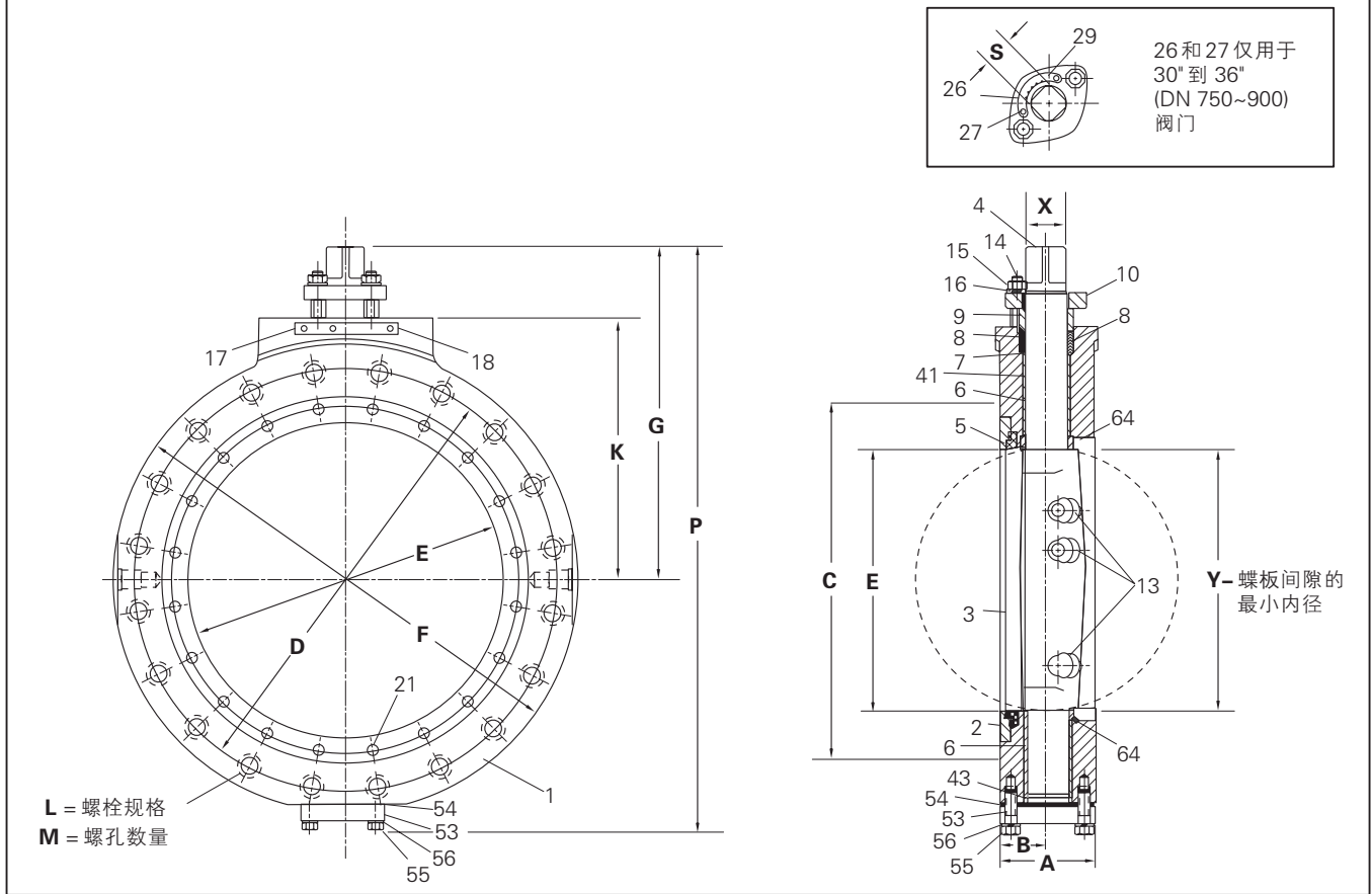
14" ~ 36" (DN350 ~ 900) 300级 830L单法兰蝶阀尺寸
