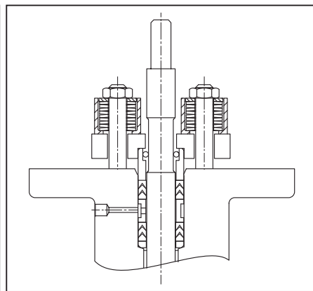
带双重填料和检测孔的动载密封(低泄漏盘根)
