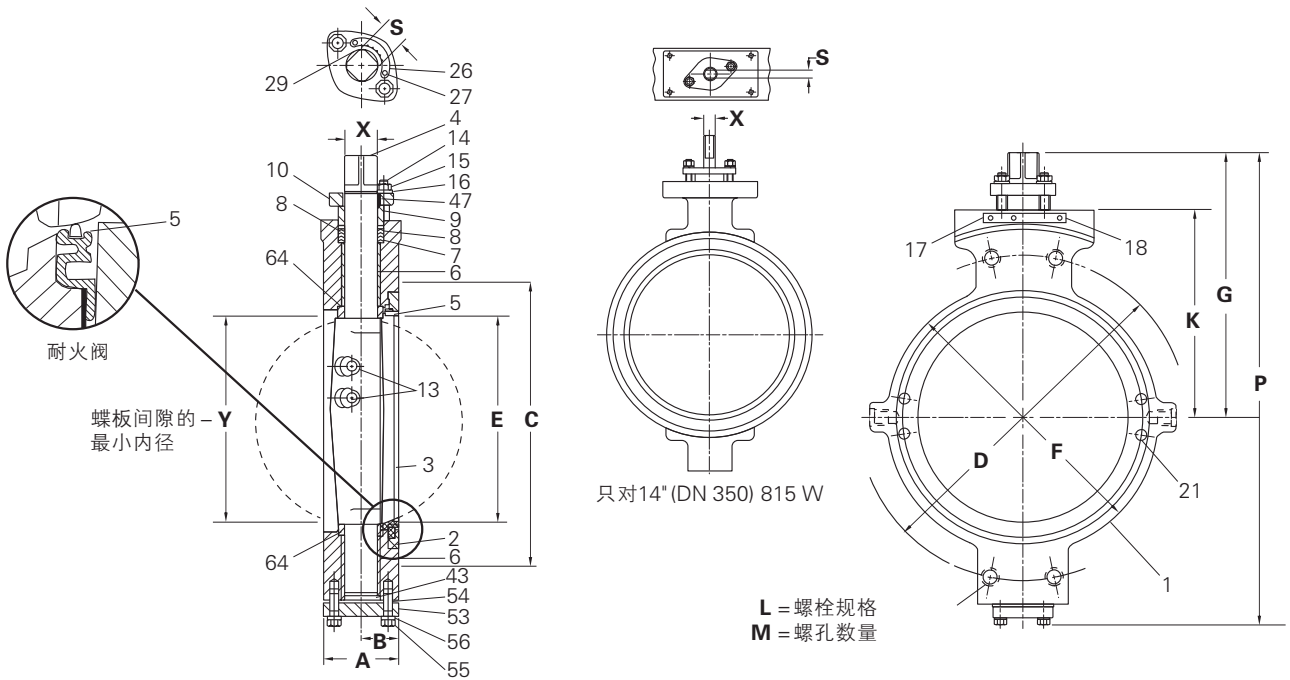
14" ~ 30" (DN350 ~ 750) 150级 815W对夹式蝶阀尺寸
